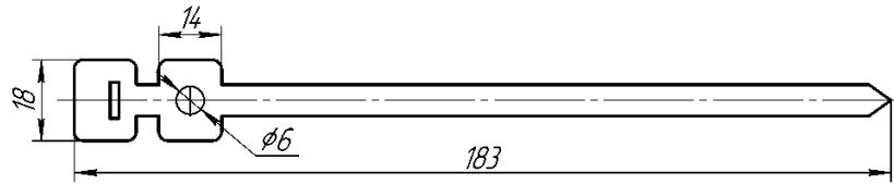
Рис. 3.3.6 Держатель ДМОУ-С
